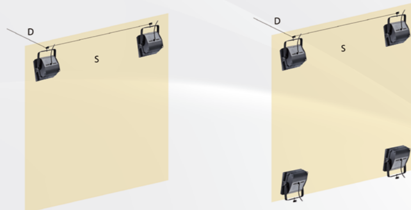
TTCY - 5100(2 qty) : S=2.0m D=2.0m
